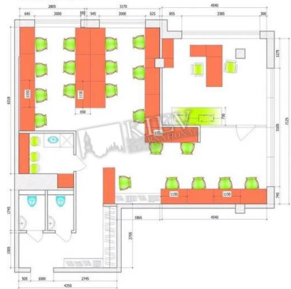
Офис Планировочный чертеж
